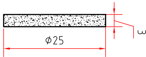
烧结金属过滤片
