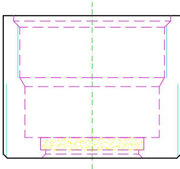
烧结金属过滤片装配位置
